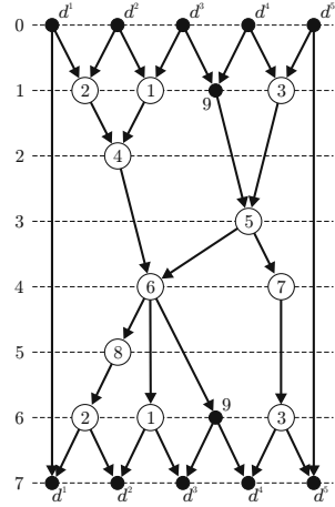
Fig. 6. Rigid (1, 1)-hierarchy
